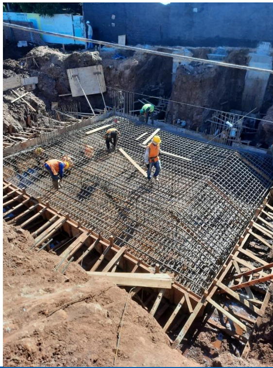
ARMADO Y HORMIGONADO DE PLATEA DE FUNDACIÓN
